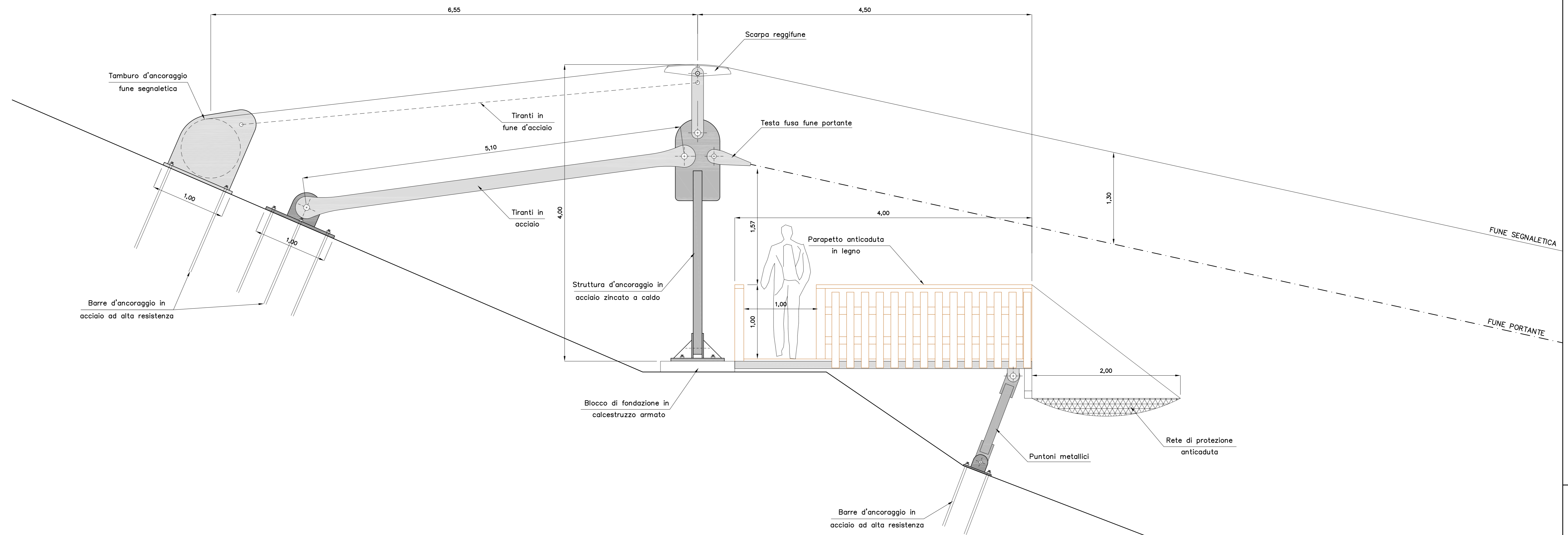
VISTA LATERALE
