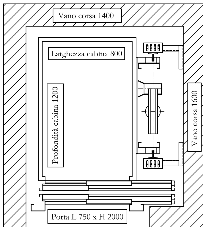
Impianto oleodinamico in taglia laterale unico accesso PORTATA 325 KG - 4 PERSONE EDIFICI PREESISTENTI
